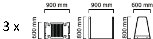
FAHRRADSTÄNDER - GROß
