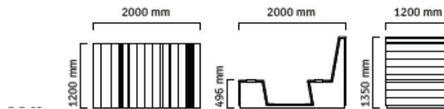
PARKLET-SITZMODUL
